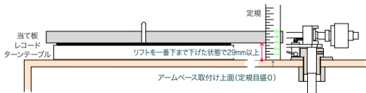
図②:アームの高さを10mmリフトアップした場合
