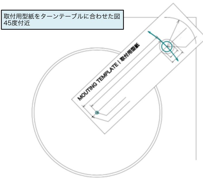
トーンアーム取付位置図
