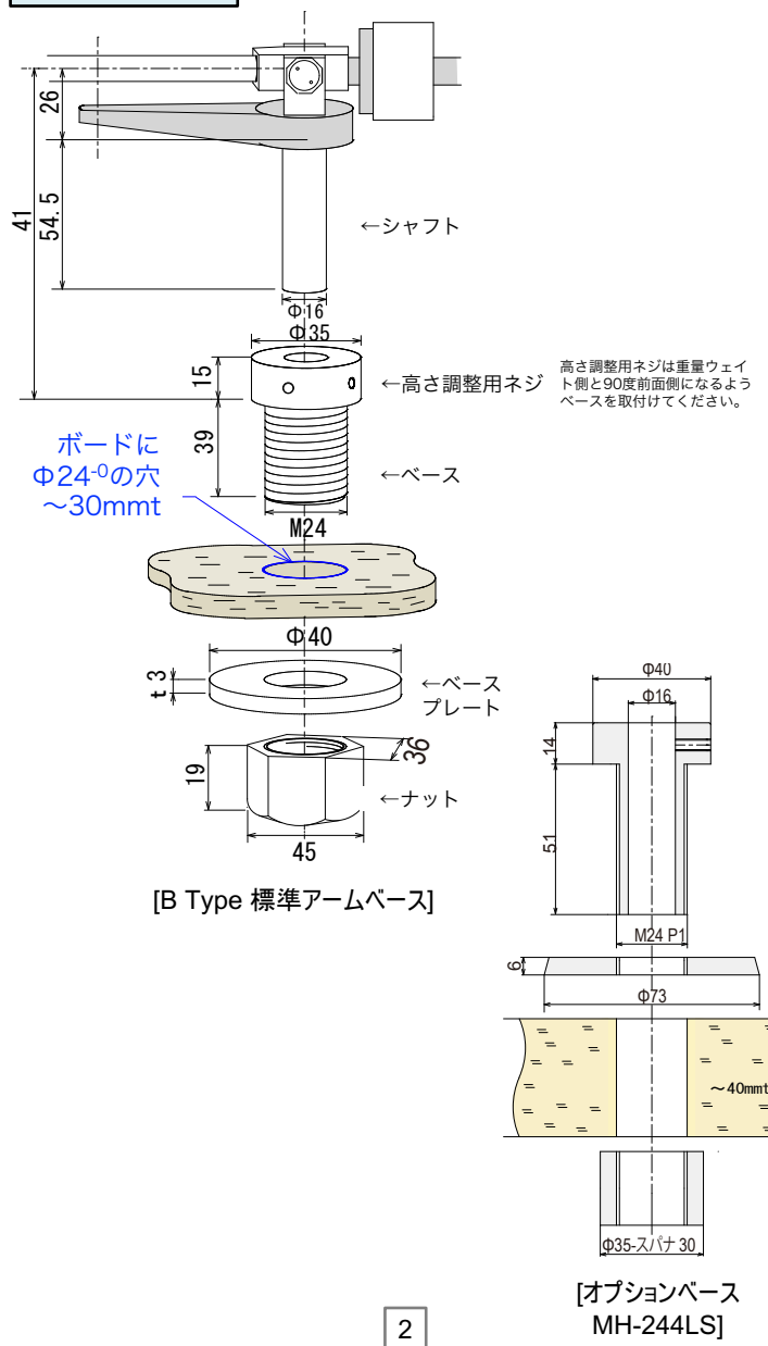
トーンアーム断面図
