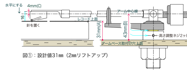
トーンアーム取付・寸法確認図 (拡大図は別紙P7,8ご参照)
