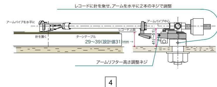
トーンアーム取付完了図 (拡大図は別紙P7,8ご参照)
