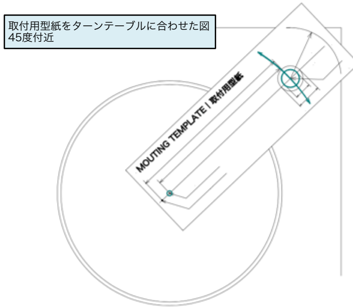
トーンアーム取付位置図
